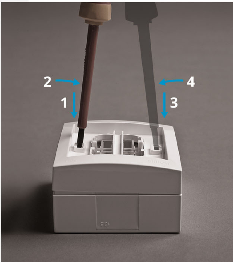
Demontaż pokryw (zwalnianie zatrząsków)
