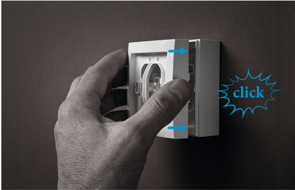
Montaż pokryw (zatrzaskiwanie)
